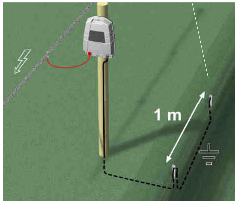
В зависимости от электропастуха и условий его работы может потребоваться от 1 до 4 заземляющих стержней Olli. Чем больше электропастух и чем суше земля, тем больше потребуется заземляющих стержней.
